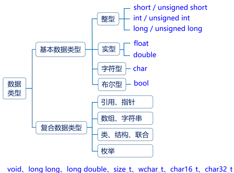
图 2.1. C++ 数据类型
