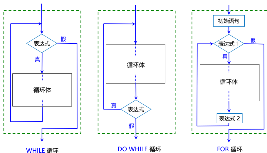
图 3.1. 三种循环示意图
