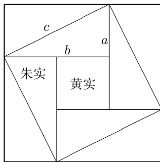
弦图
