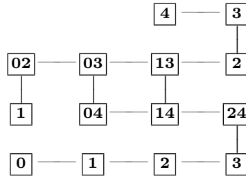
\mathfrak{M}_4
