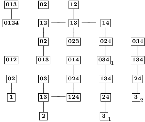
\mathfrak{M}_{23}
