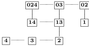
\mathfrak{M}_8
