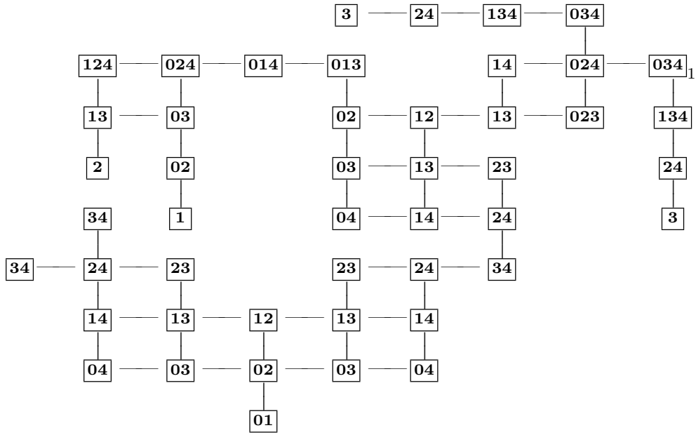
\mathfrak{M}_{15}
