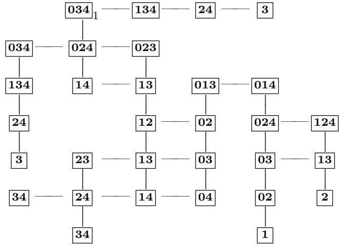
\mathfrak{M}_{13}
