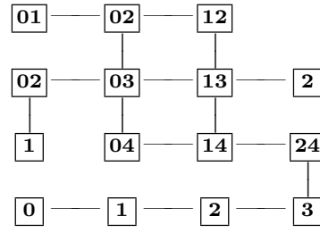
\mathfrak{M}_5
